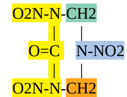
Keto-RDX
