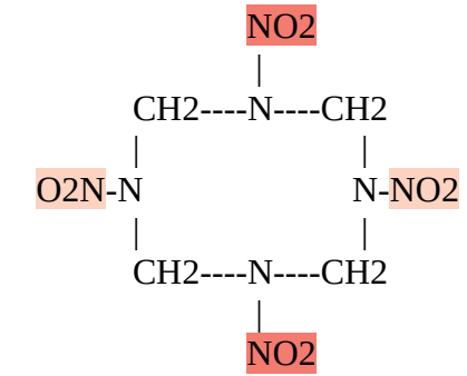
HMX
